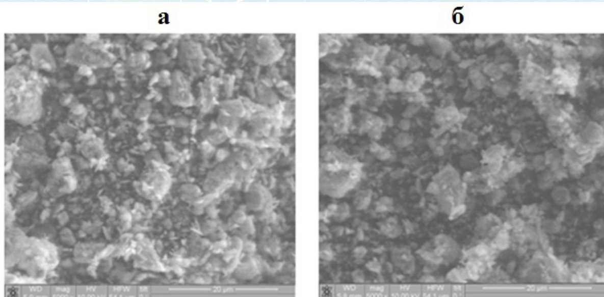
3-расм. Бентонитнамунасининг 90минут (а) ва 100минут (б) механик қайта ишлангандан кейинги микрофотографияси
