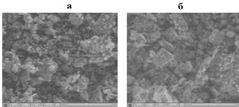
1-расм. Бентонитнинг микрофотографияси а)намунанинг дастлабки ва б)30минут механик қайта ишлангандан кейинги микрофотографияси
