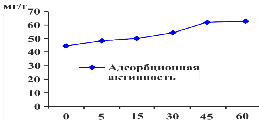
4-расм. Адсорбцион фаоллиқнинг ўзгаришини механик қайта ишлаш вақтига боғлиқлигининг ўзгариш динамикаси.
