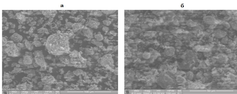
1-расм. Бентонитнинг микрофотографияси а)намунанинг дастлабки ва б)30минут механик қайта ишлангандан кейинги микрофотографияси
