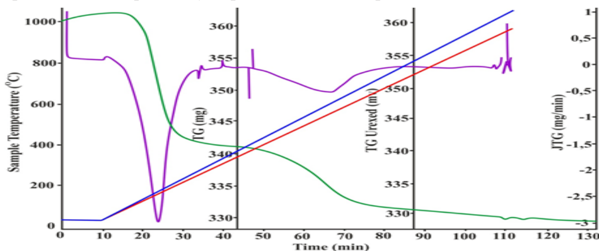
5-расм. Навбахордан топилган бентонитнинг дериватограммаси.
